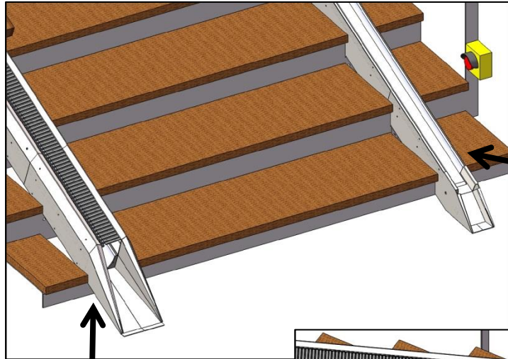
Lopende band/ tandriem (van beneden naar boven)
